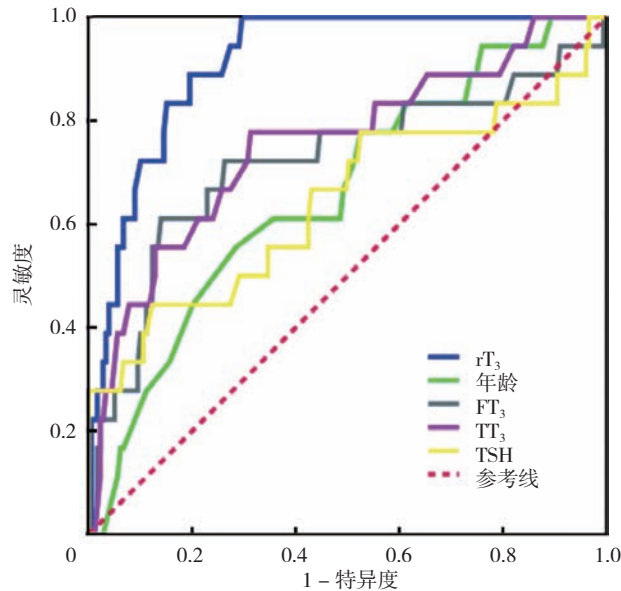
注: rT 3 =反三碘甲状腺原氨酸, FT 3 =游离三碘甲状腺原氨酸, TT 3 =总三碘甲状腺原氨酸, TSH=促甲状腺激素。 图1 FT 3 、TT 3 、TSH、rT 3 和年龄预测心力衰竭患者住院期间死亡的ROC曲线
